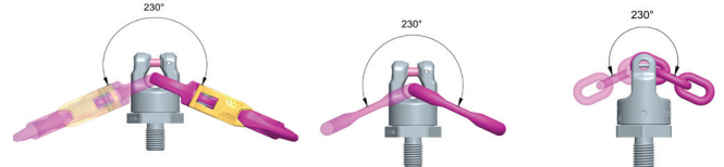
Abb. 2: Schwenkbereich PP-S/PP-B/PP-VIP
